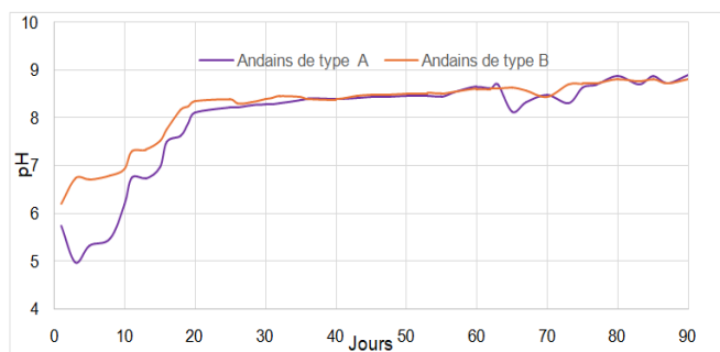
Figure 4. Évolution moyenne du pH dans les deux types d'andains
