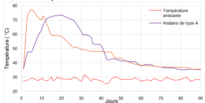
Figure 3. Évolution moyenne de la température dans les deux types d'andains
